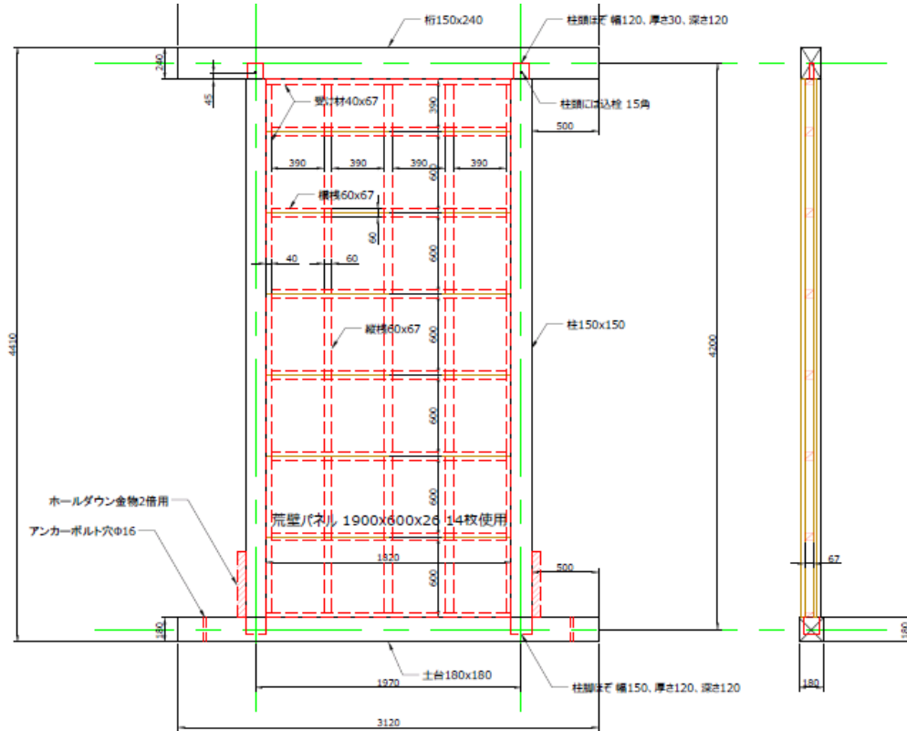
図 耐震補強壁
